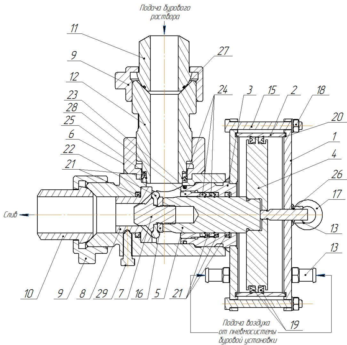
Схема ДЗУ-400, 530
