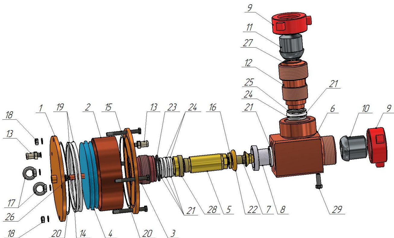
Схема сборки дроссельно-запорного устройства 400, 530
